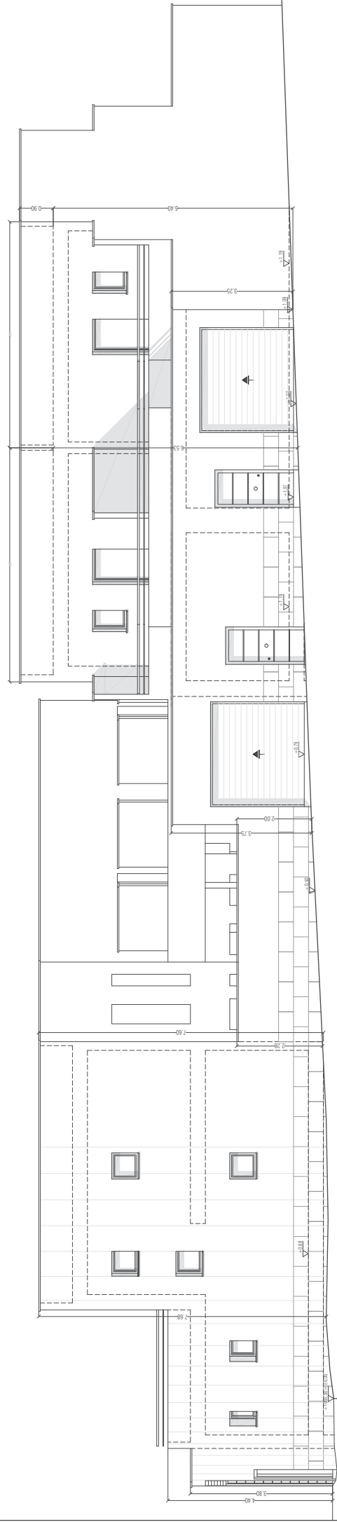
ALZADO C/Cº DE ESPIRDO
